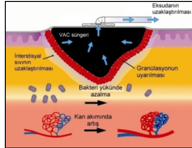
Resim 2. Vakum yardımcı kapama şematik çalışma şekli
